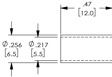
FERRULE
