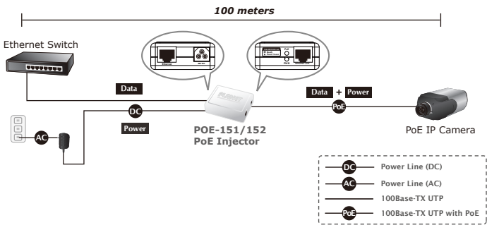
Bild 3: Verbindung zum IEEE 802.3af Gerät
