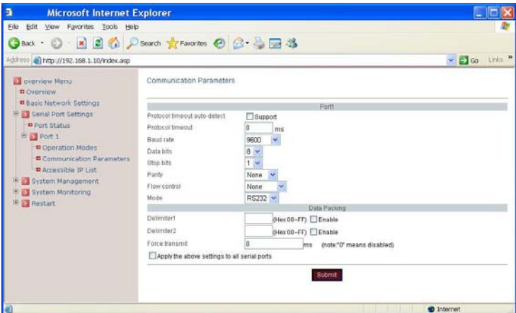
Fig 12. Communication Parameters
