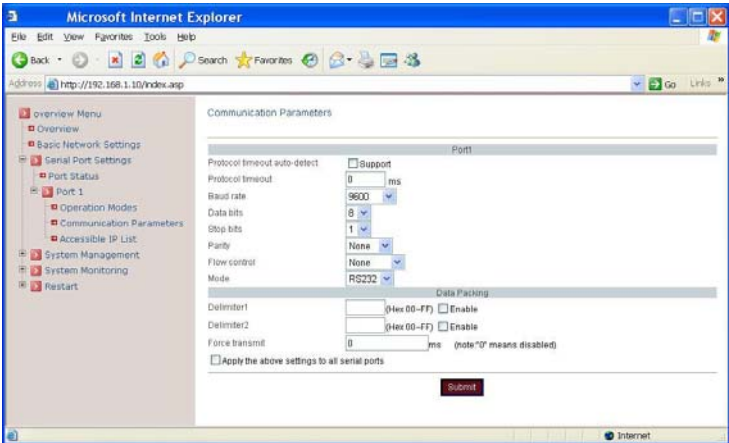
Fig 19. Communication Parameters
