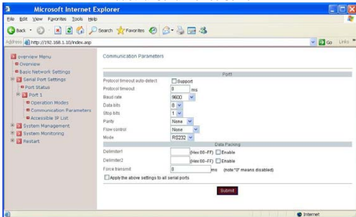
Fig 17. Communication Parameters
