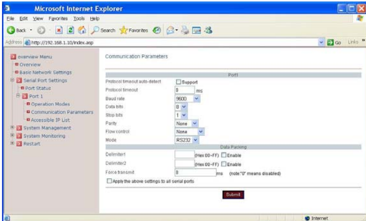
Fig 9. Communication Parameters
