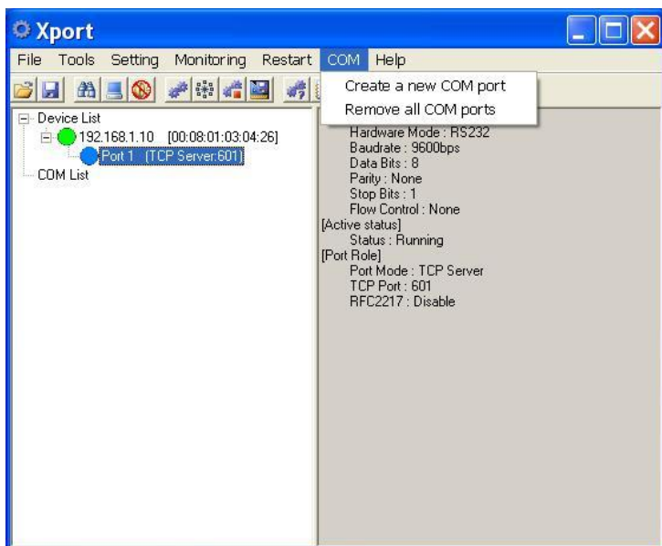
Fig 92. COM
