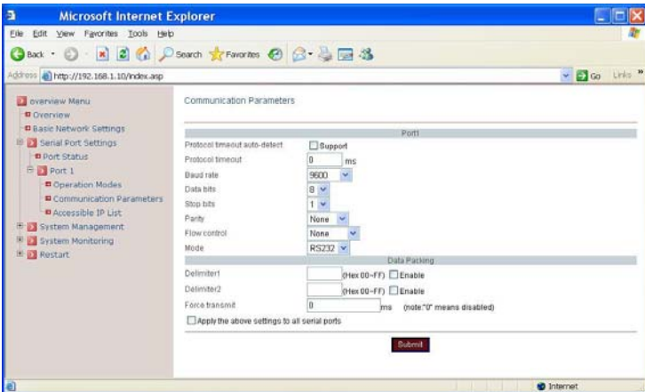
Fig 14. Communication Parameters
