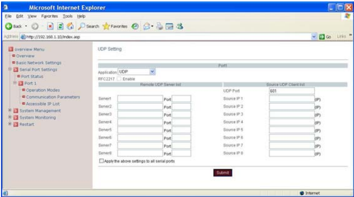
Fig 18. UDP Setting
