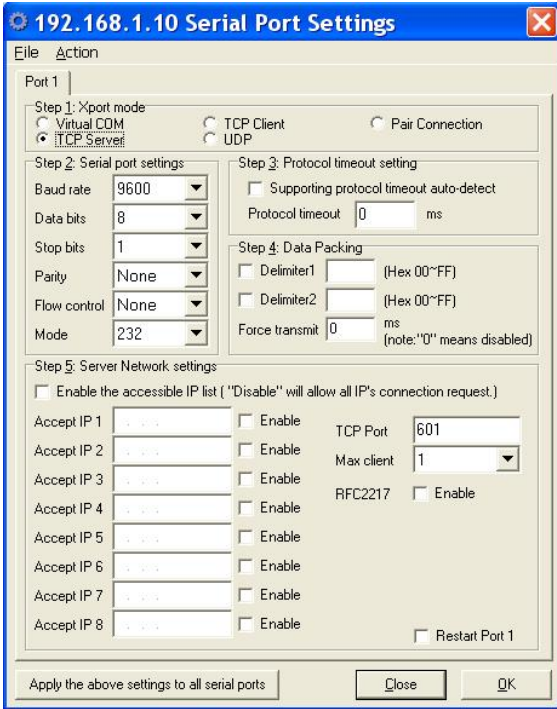
Fig 77. TCP Server
